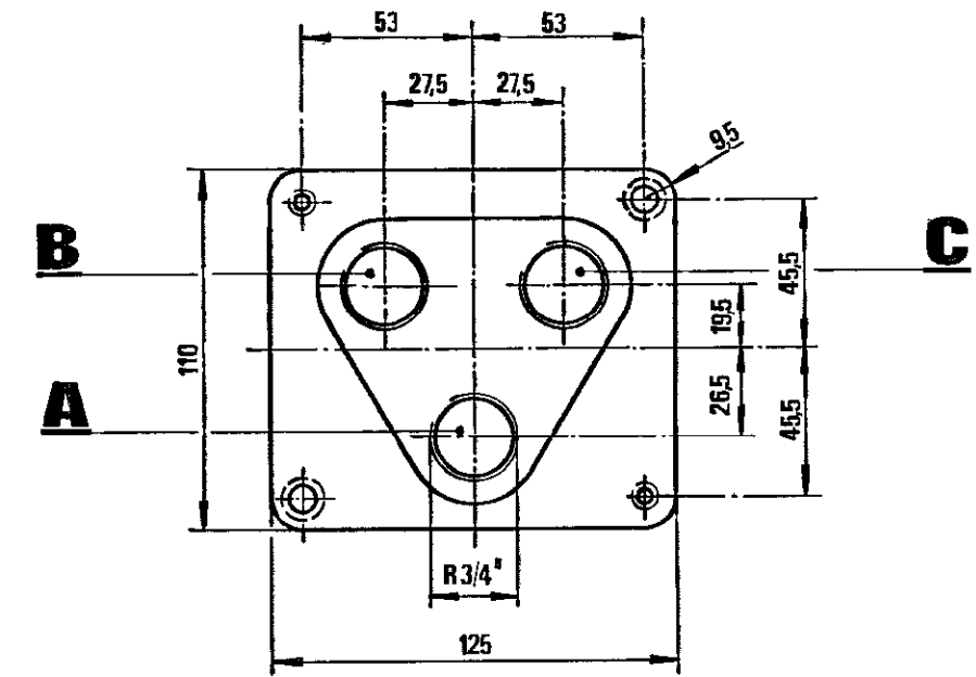
Ansicht A
